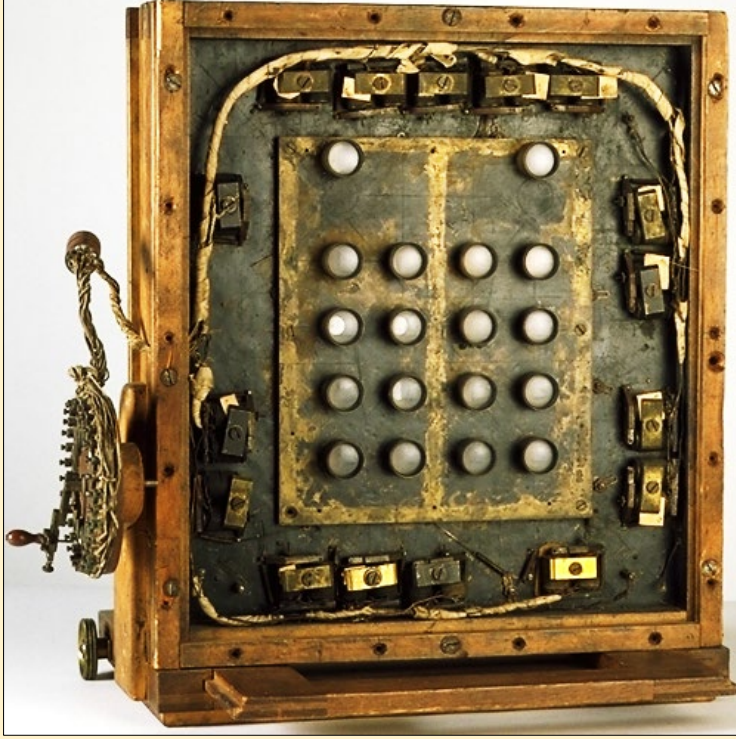
16 OBJEKTİFLİ KAMERA LOUIS LE PRİNCE (TALİP KOÇ ARŞİVİ)
